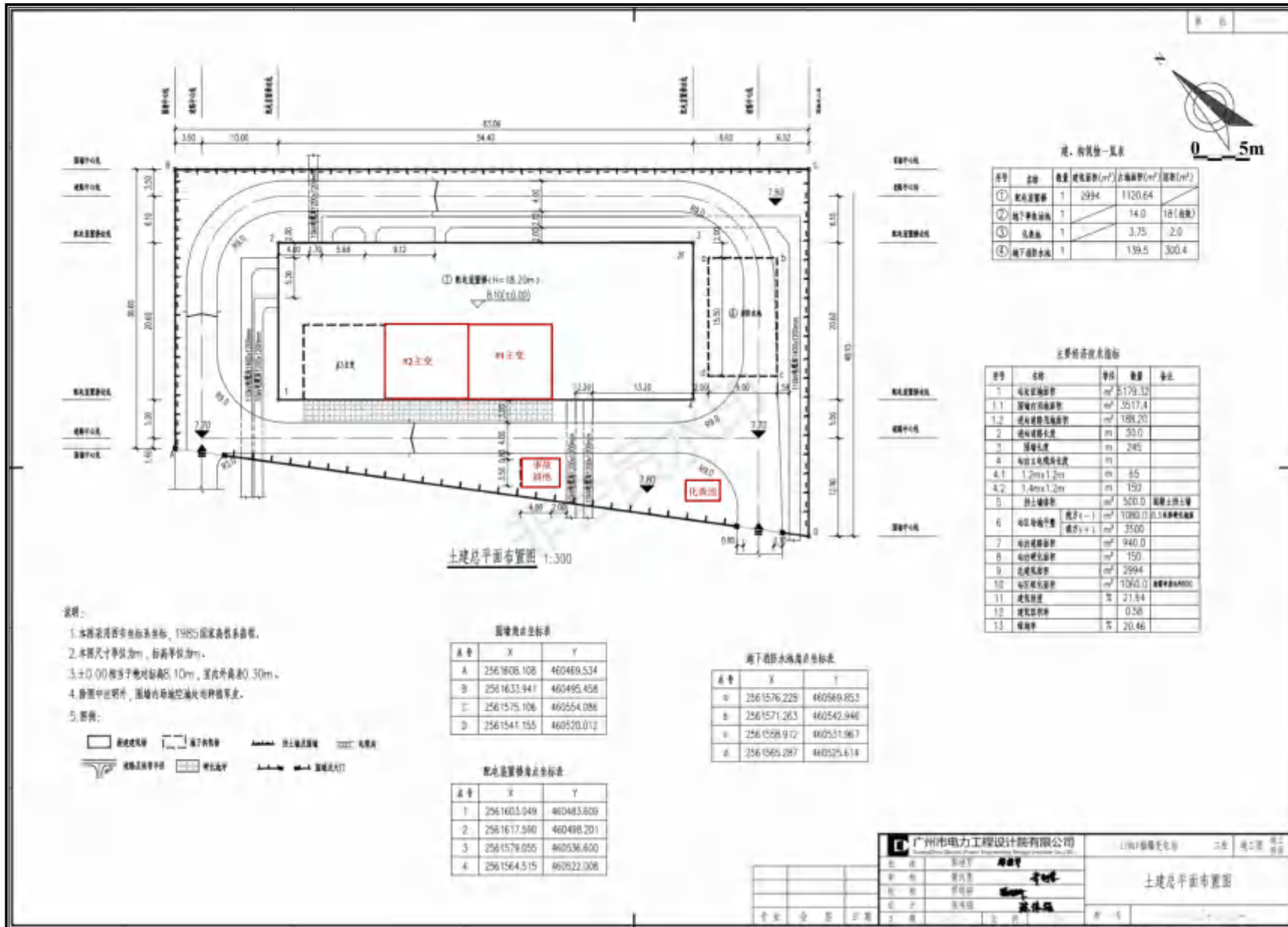
附图 4 110kV 福耀变电站总平面布置图
