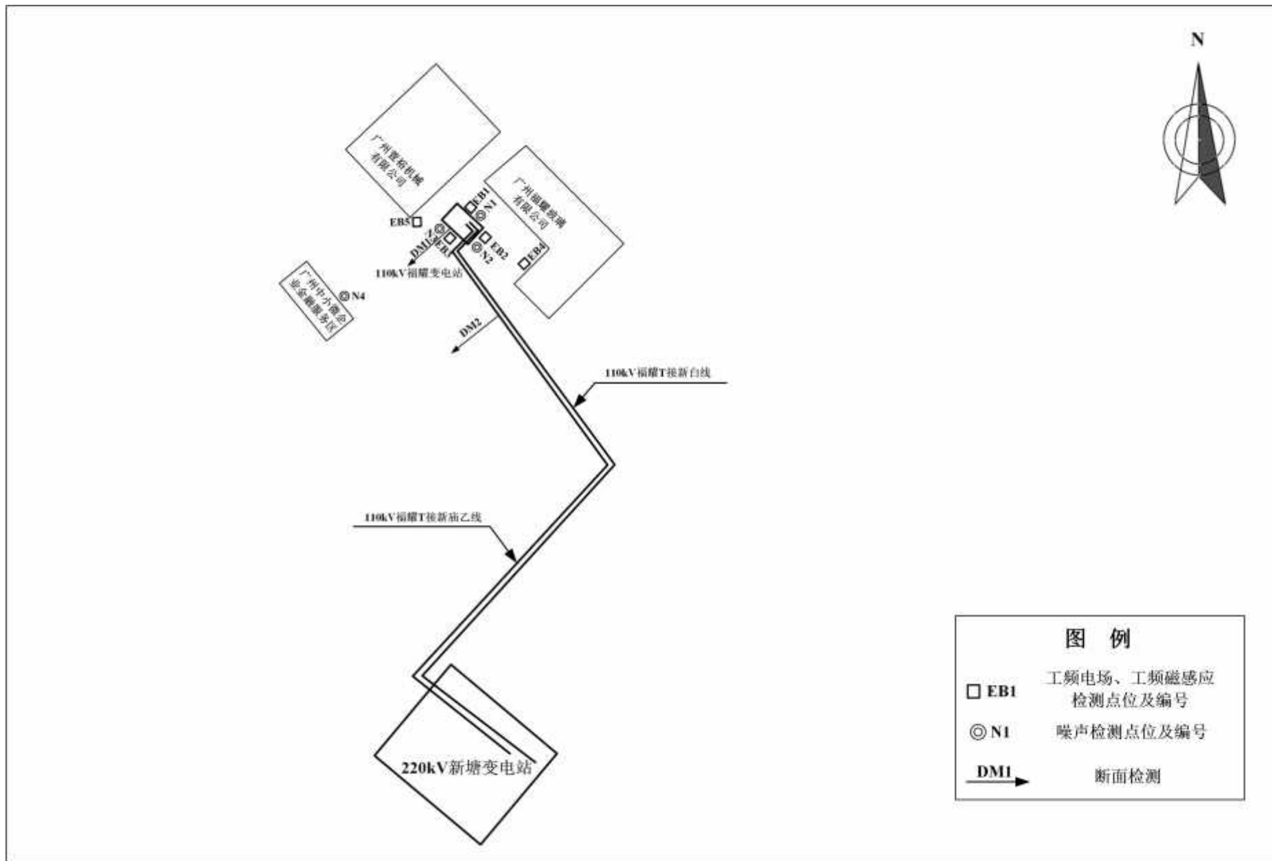
附图 5 110kV 福耀输变电工程监测点位图
