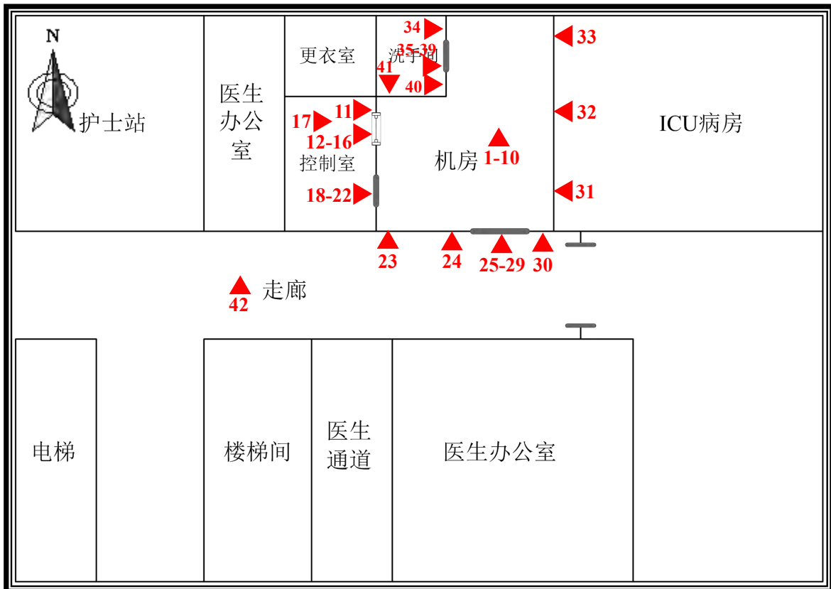
图 7-2 DSA 机房防护效果检测点位示意图 (▲ 检测点位)
