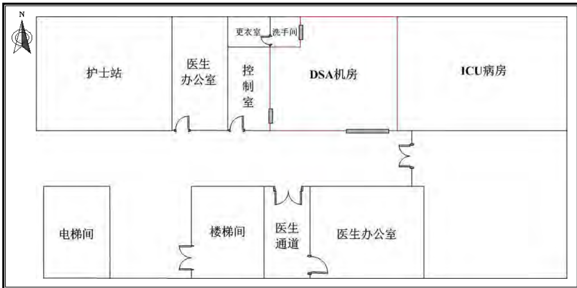
图 3-3 DSA 机房周边平面布局图
